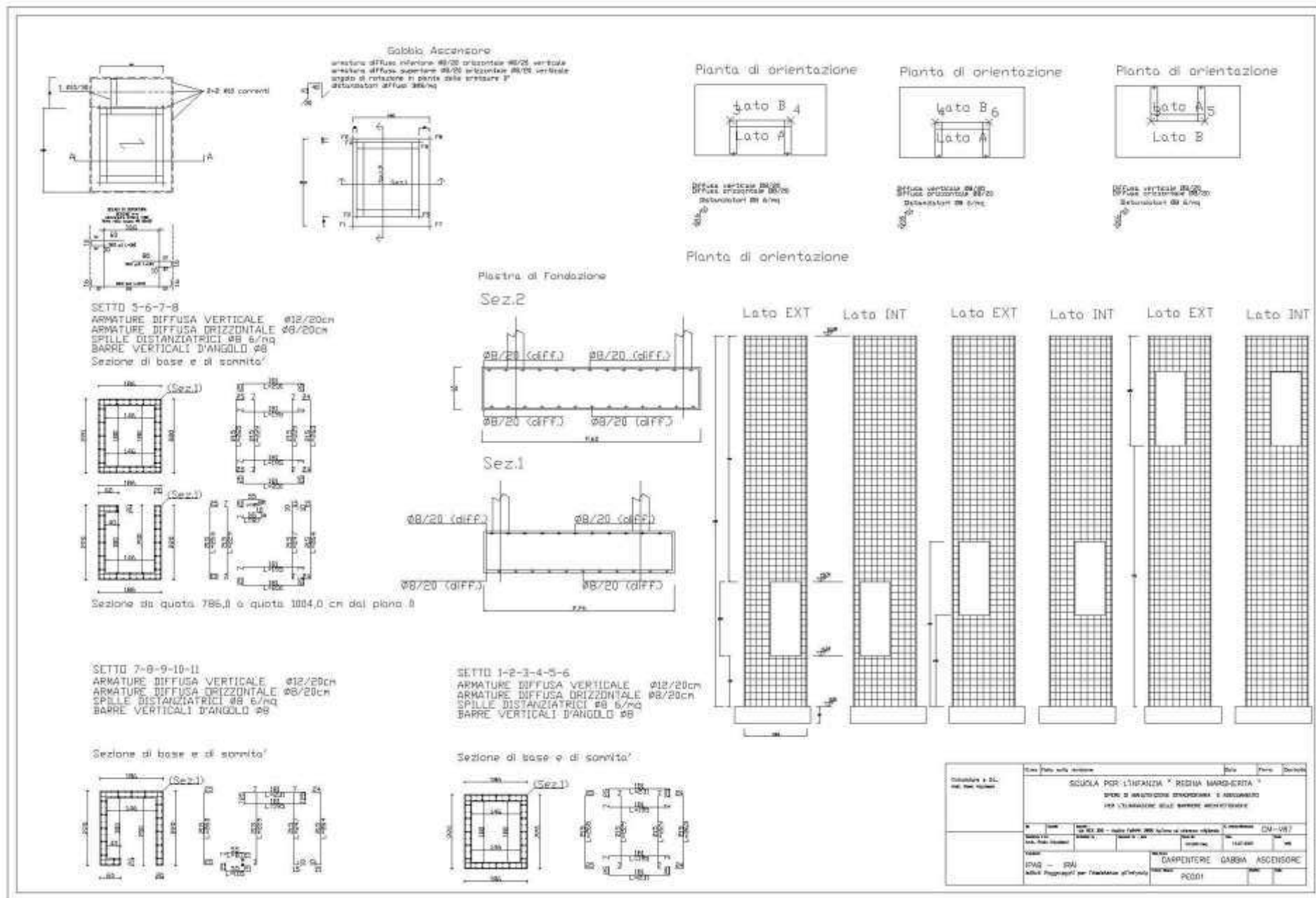
Roma – San Lorenzo – Scuola per l'infanzia "Regina Margherita" Adeguamento Barriere architettoniche – Realizzazione Ascensore Progetto delle strutture
