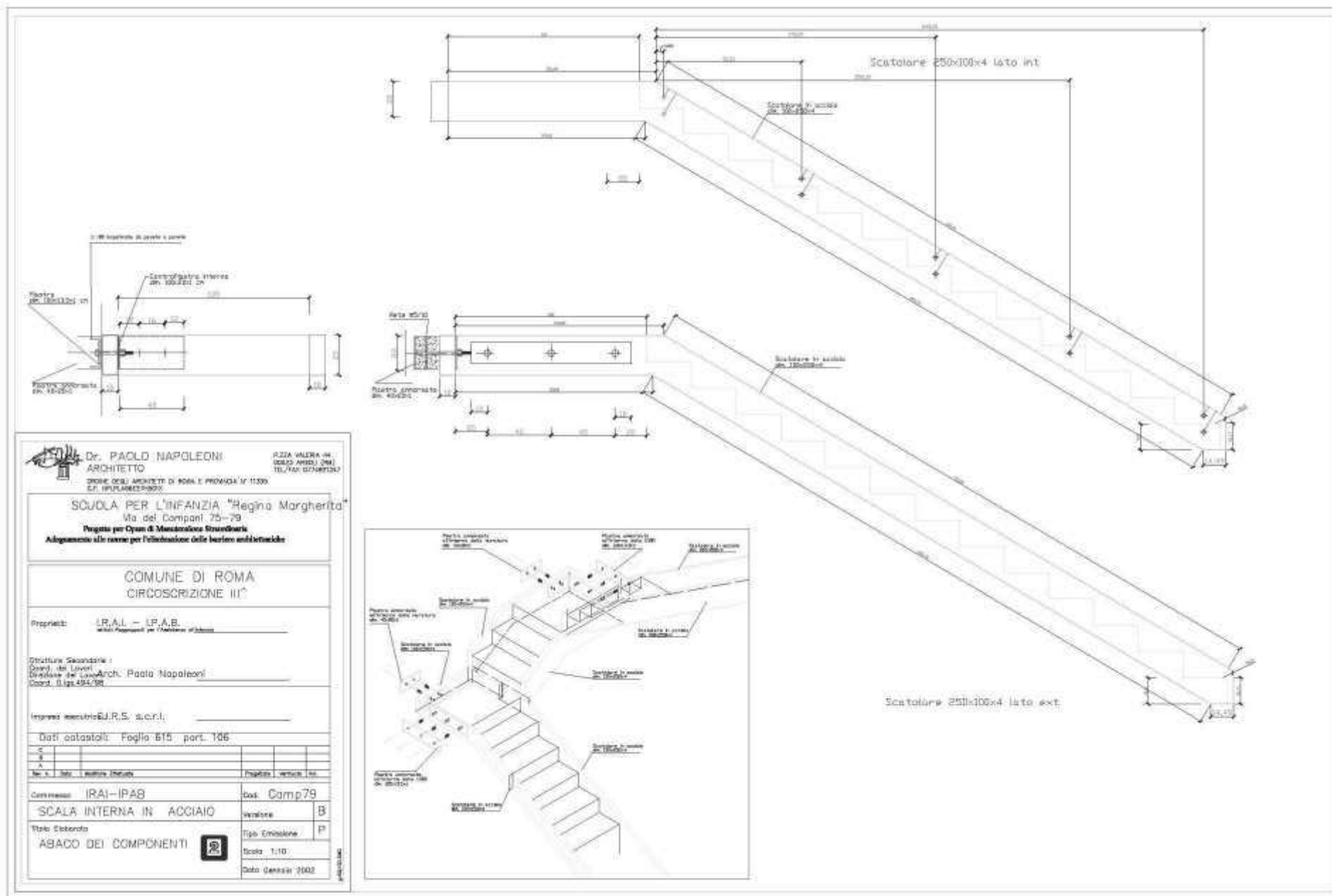
Roma – San Lorenzo – Scuola per l'infanzia “Regina Margherita” Adeguamento Barriere architettoniche – Realizzazione Nuova scala interna – Abaco dei componenti
