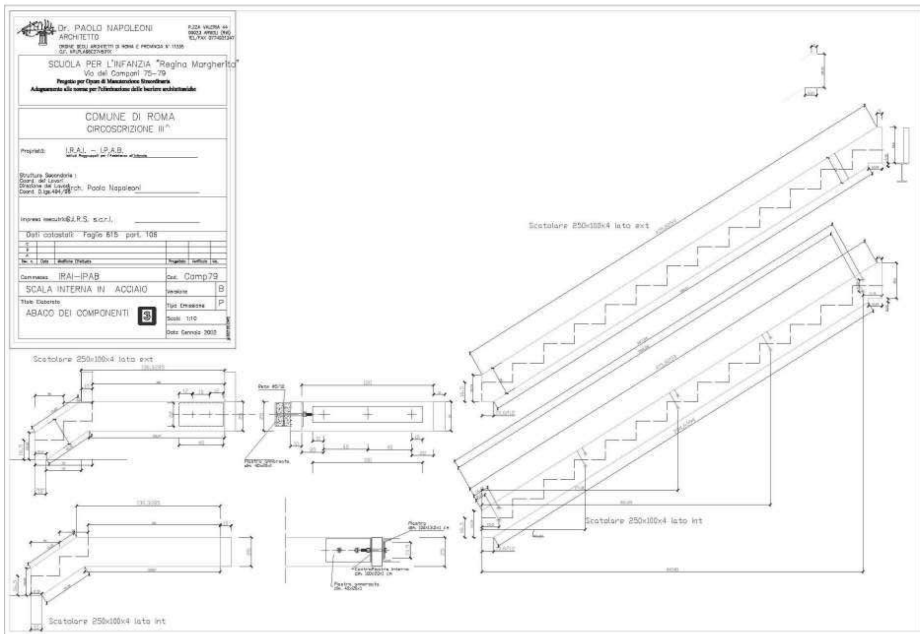
Roma – San Lorenzo – Scuola per l’infanzia “Regina Margherita” Adeguamento Barriere architettoniche – Realizzazione Nuova scala interna – Abaco dei componenti.
