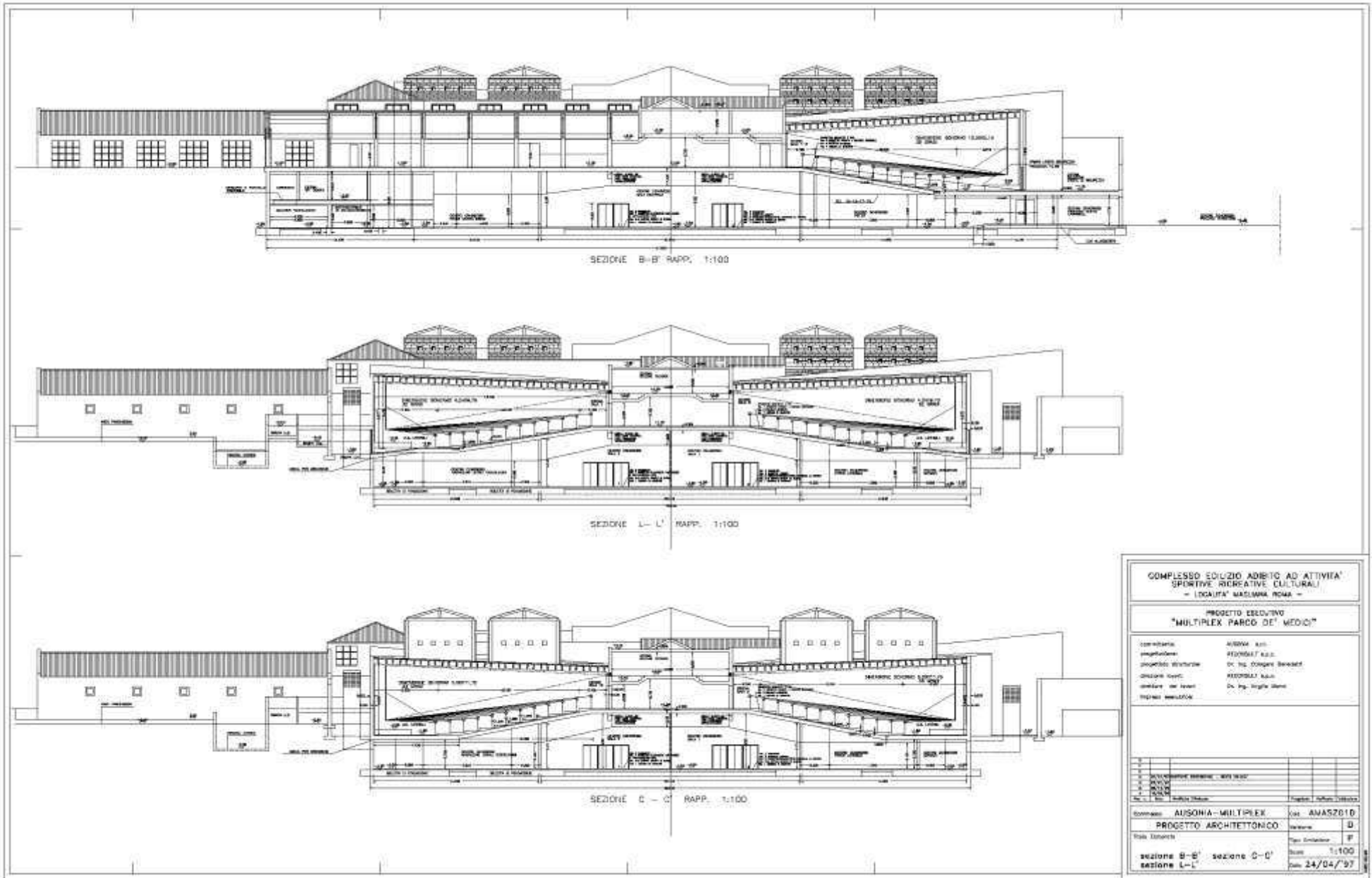
Roma – Magliana - Complesso edilizio adibito ad attività culturali – Multiplex Parco de Medici.
