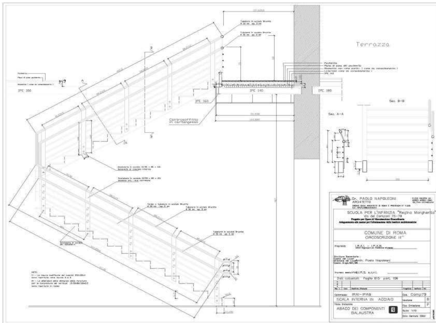
Roma – San Lorenzo – Scuola per l'infanzia “Regina Margherita” Adeguamento Barriere architettoniche – Realizzazione Nuova scala interna – Abaco dei componenti della balaustra
