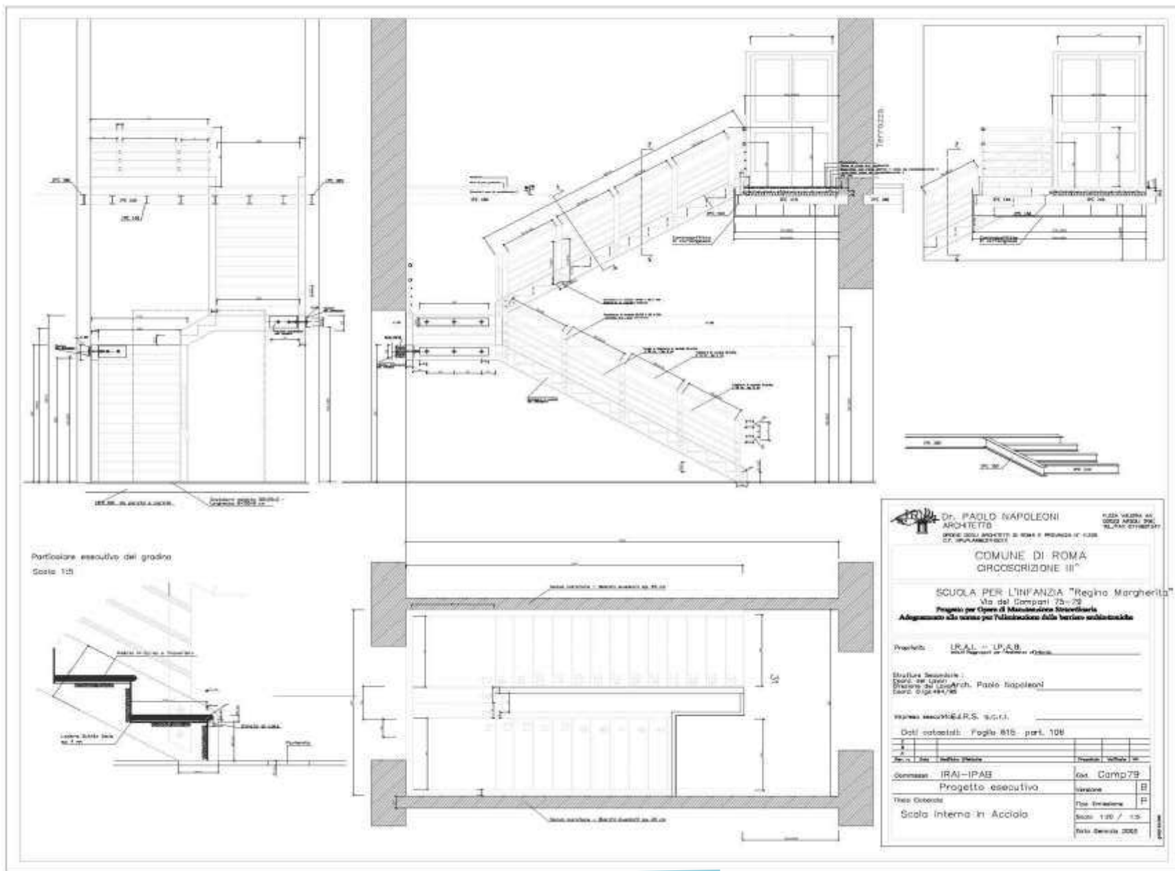
Roma – San Lorenzo – Scuola per l’infanzia “Regina Margherita” Adeguamento Barriere architettoniche – Realizzazione Nuova scala interna - Progetto delle strutture.
