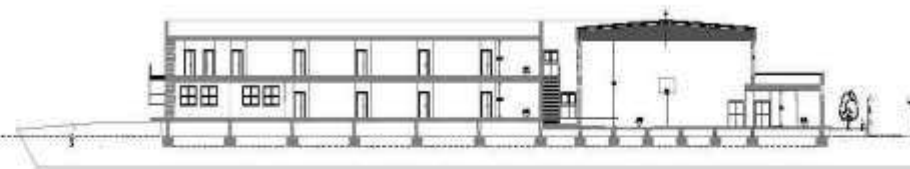
SEZIONE A-A'
