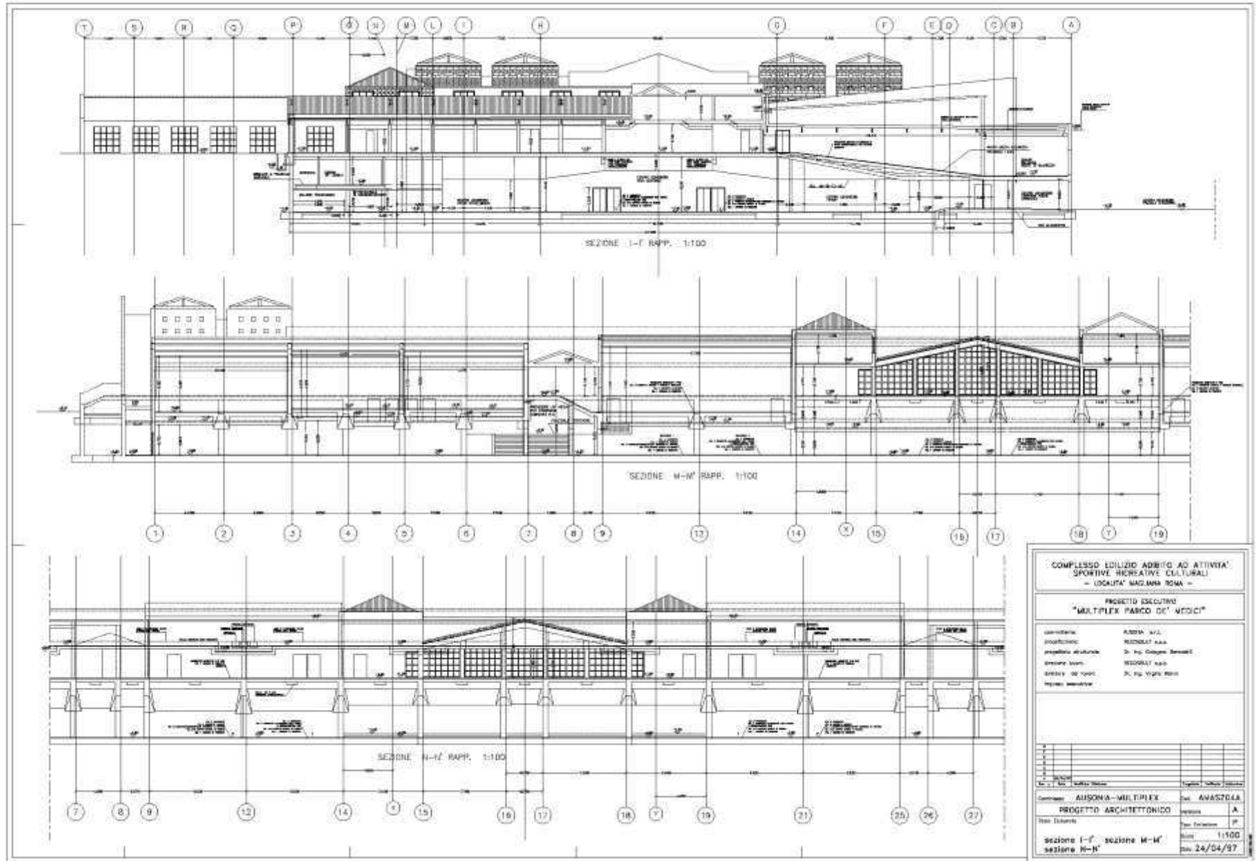
Roma – Magliana - Complesso edilizio adibito ad attività culturali – Multiplex Parco de Medici.
