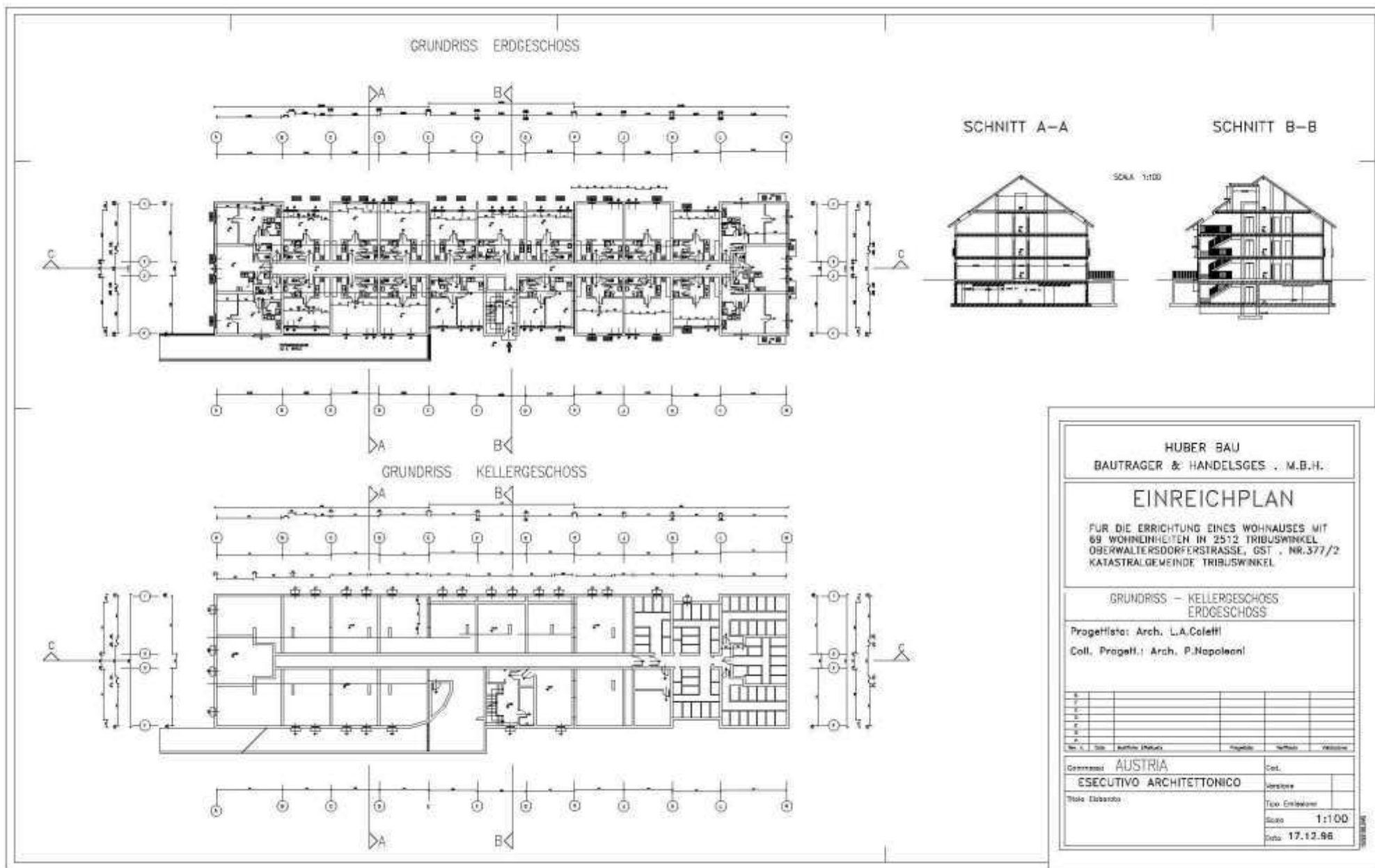
Austria – Tribuswinkel – Alloggi per anziani ad alta efficienza energetica. Soc. AEDIFICA S.r.L.– Progetto Definitivo
