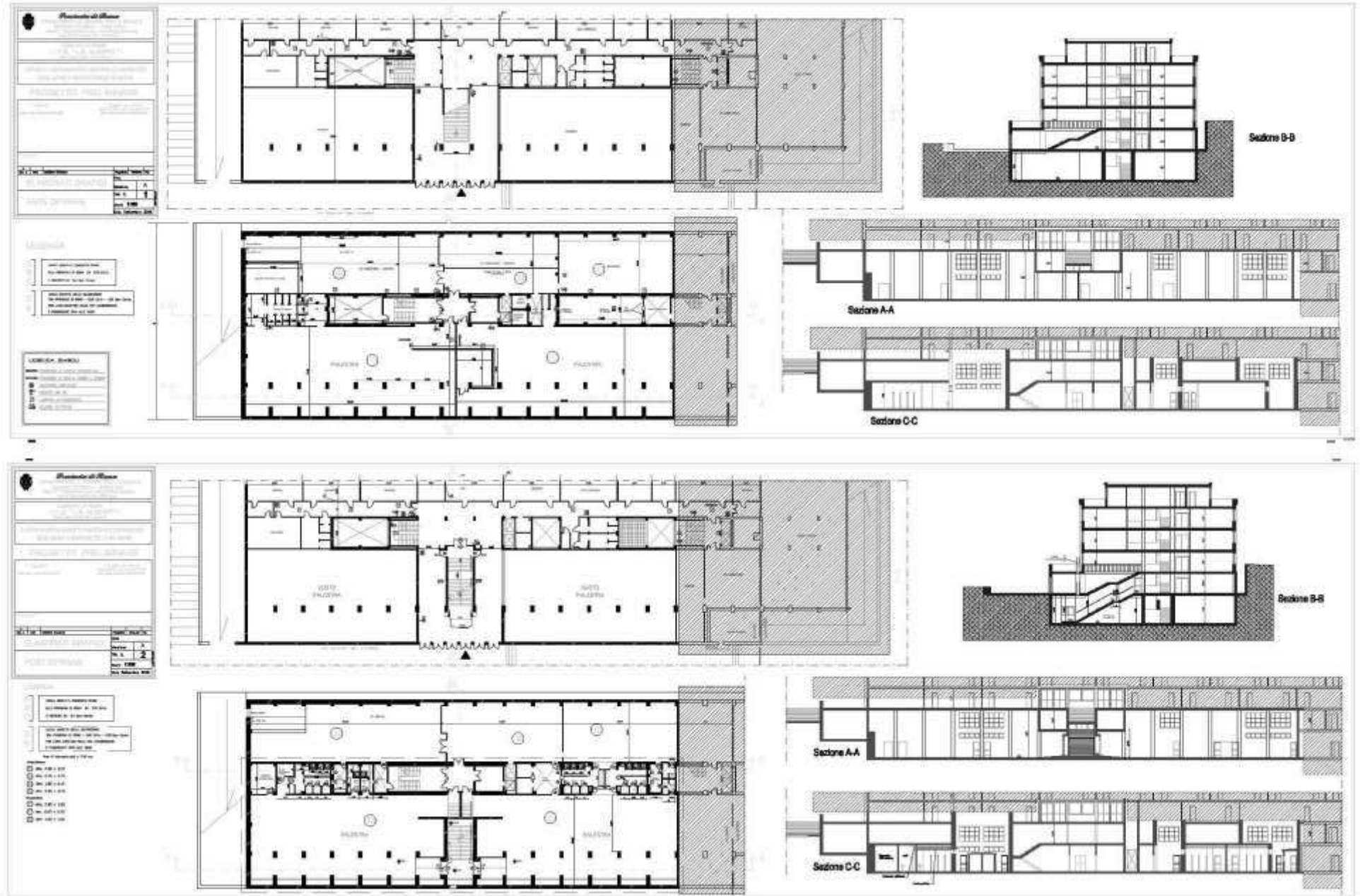
Istituto per Geometri L.B.Alberti – Ripristino della funzionalità delle Palestre e dei servizi annessi.
