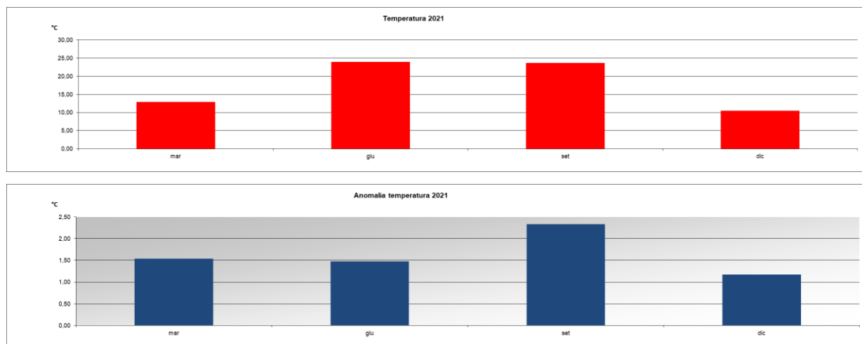
Fig. 3.1 Distribuzione delle temperature atmosferiche e anomalie della temperatura atmosferica nel 2021
