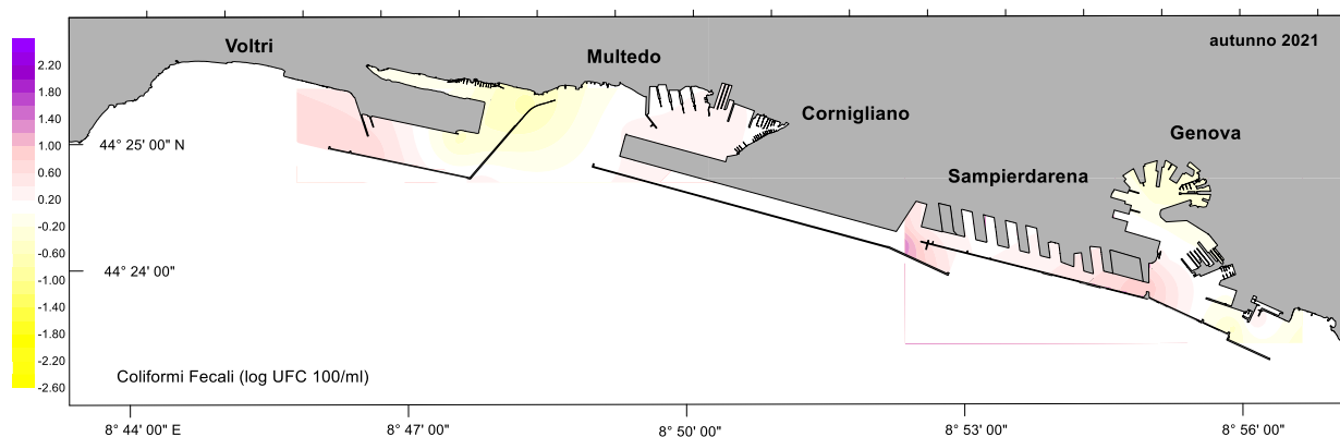
Fig. 3.9 Distribuzione spaziale delle anomalie dei coliformi fecali nel 2021
