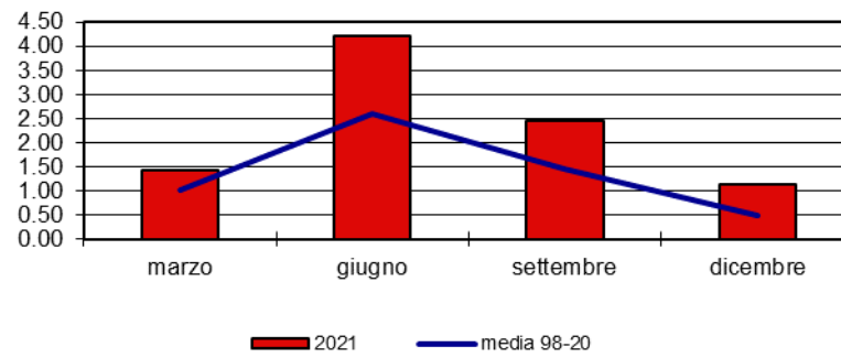
Coliformi fecali (MPN/100 ml)
