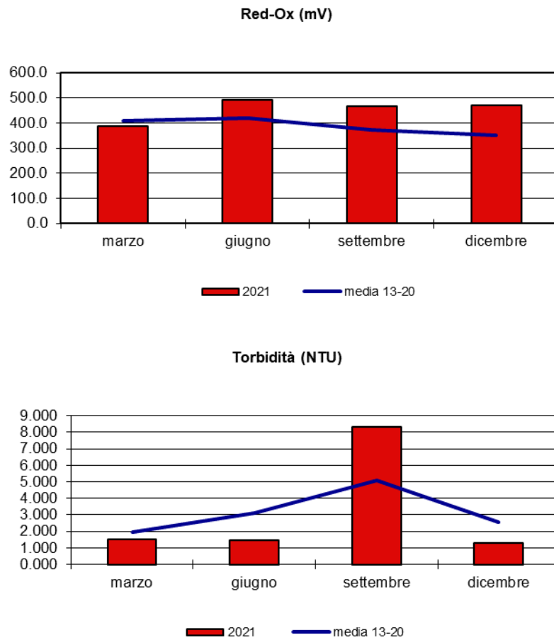
Fig. 3.20 Evoluzione annuale dei parametri provenienti dal monitoraggio 2021 rispetto alla media calcolata nel periodo 1998-2020 (2013-2020 per pH, Red-Ox e torbidità). (stazione 34)
