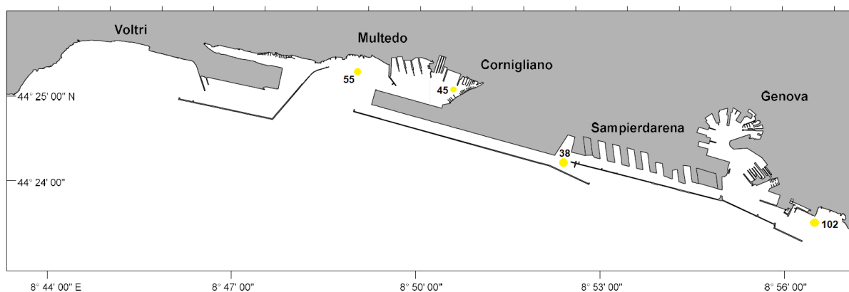
Fig. 2.3 Punti di campionamento dei sedimenti marini dell'anno 2021.
