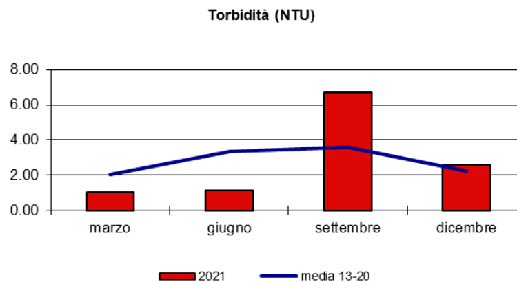
Fig. 3.18 Evoluzione annuale dei parametri provenienti dal monitoraggio 2021 rispetto alla media calcolata nel periodo 1998-2020 (2013-2020 per pH, Red-Ox e torbidità). (stazione 104)
