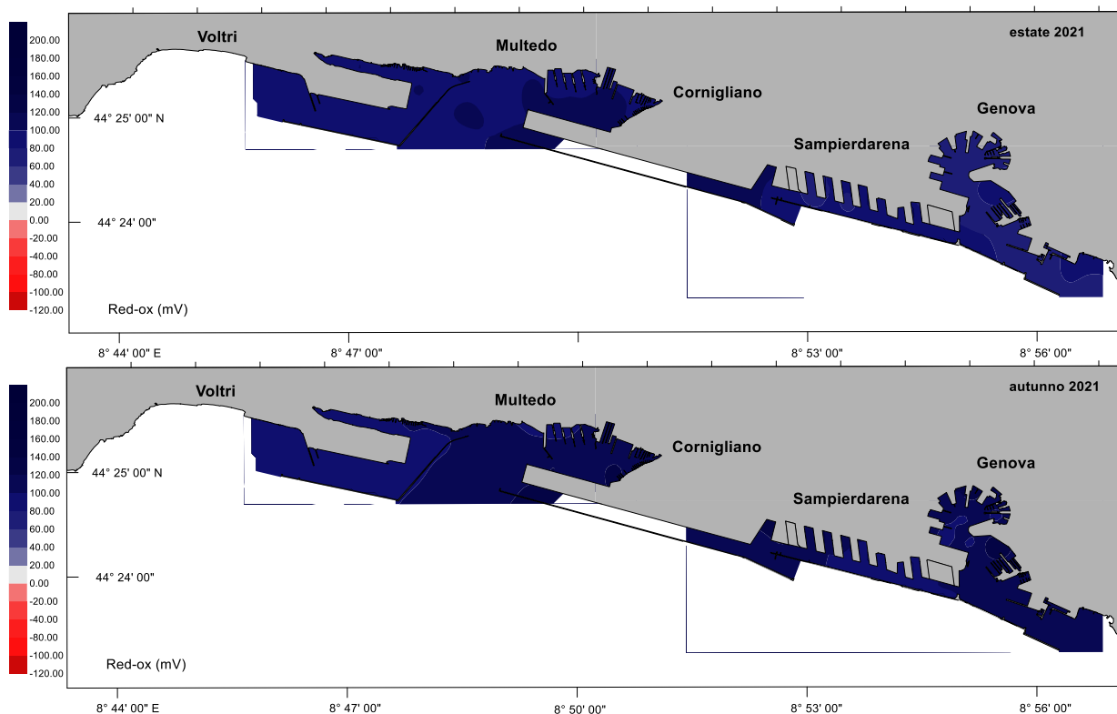
Fig. 3.11 Distribuzione spaziale delle anomalie di potenziale Red-Ox nel 2021
