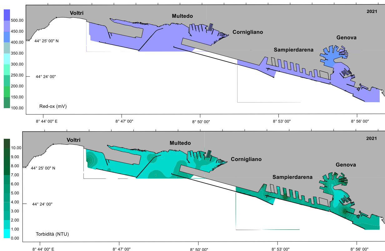
Fig. 3.13 Distribuzioni spaziali (media annuale) di temperatura, salinità, ossigeno disciolto, clorofilla-a, ammoniaca, coliformi fecali, pH, potenziale Red-Ox e torbidità.
