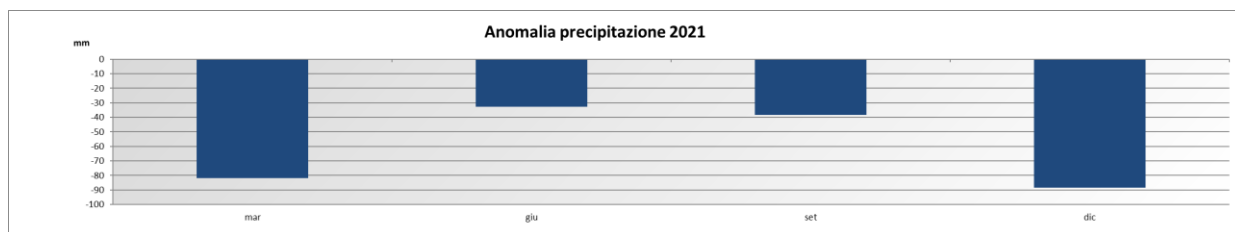
Fig. 3.2 Distribuzione delle precipitazioni, dei giorni di pioggia e anomalie delle precipitazioni nel 2021
