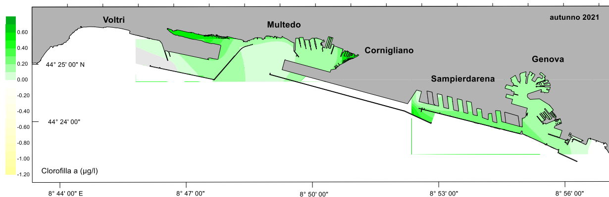
Fig. 3.7 Distribuzione spaziale delle anomalie della clorofilla a nel 2021
