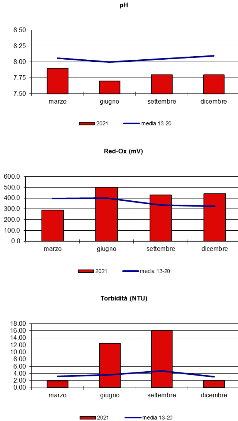
Fig. 3.16 Evoluzione annuale dei parametri provenienti dal monitoraggio 2021 rispetto alla media calcolata nel periodo 1998-2020 (2013-2020 per pH, Red-Ox e torbidità). (stazione 10)
