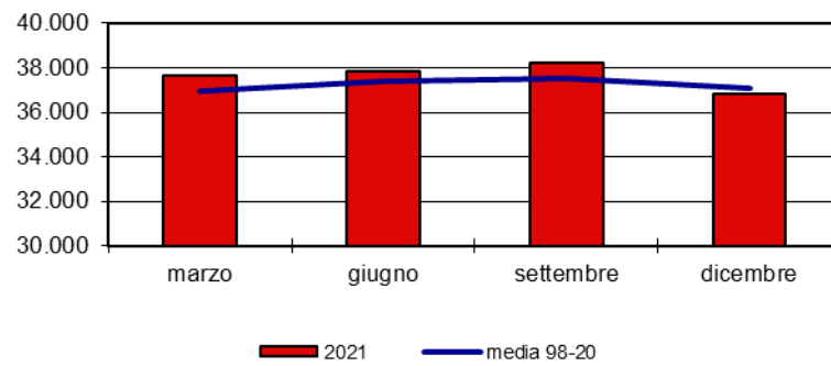
Ossigeno disciolto (% sat)
