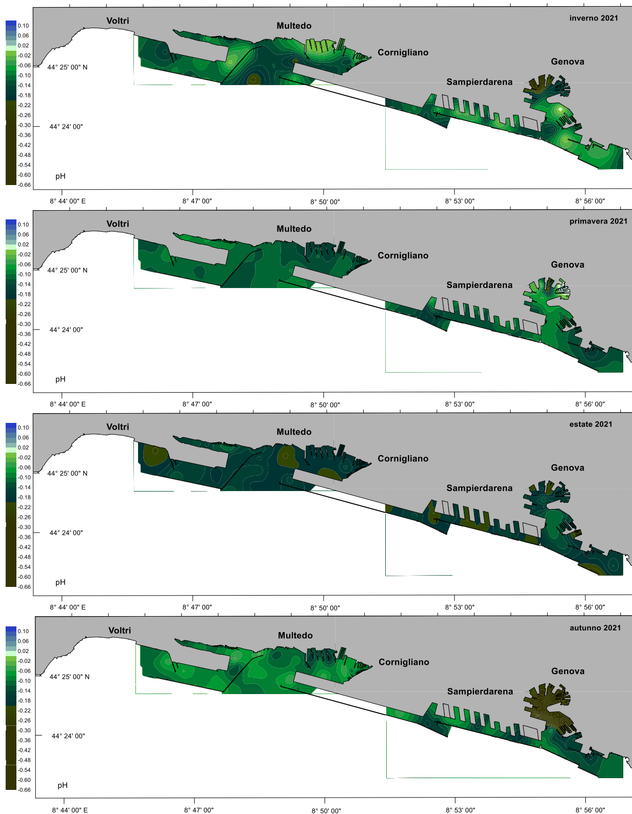
Fig. 3.10 Distribuzione spaziale delle anomalie di pH nel 2021
