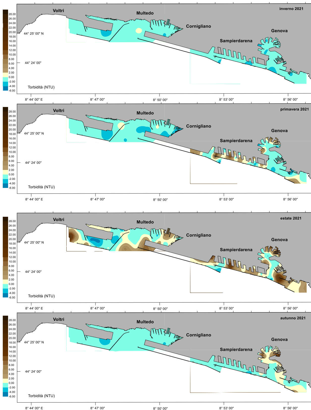
Fig. 3.12 Distribuzione spaziale delle anomalie di torbidità nel 2021
