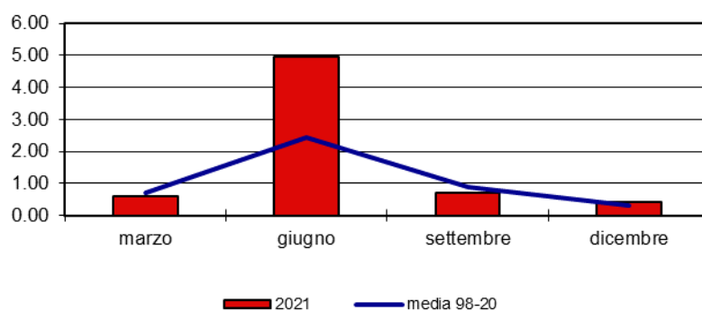
Coliformi fecali (MPN/100 ml)
