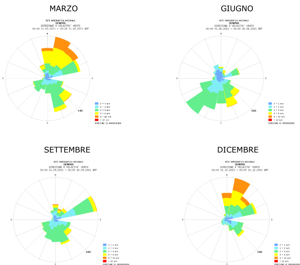
Fig. 3.3 Distribuzione dei venti nel 2021
