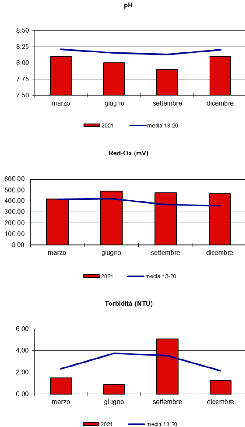
Fig. 3.22 Evoluzione annuale dei parametri provenienti dal monitoraggio 2021 rispetto alla media calcolata nel periodo 1998-2020 (2013-2020 per pH, Red-Ox e torbidità). (stazione 43)
