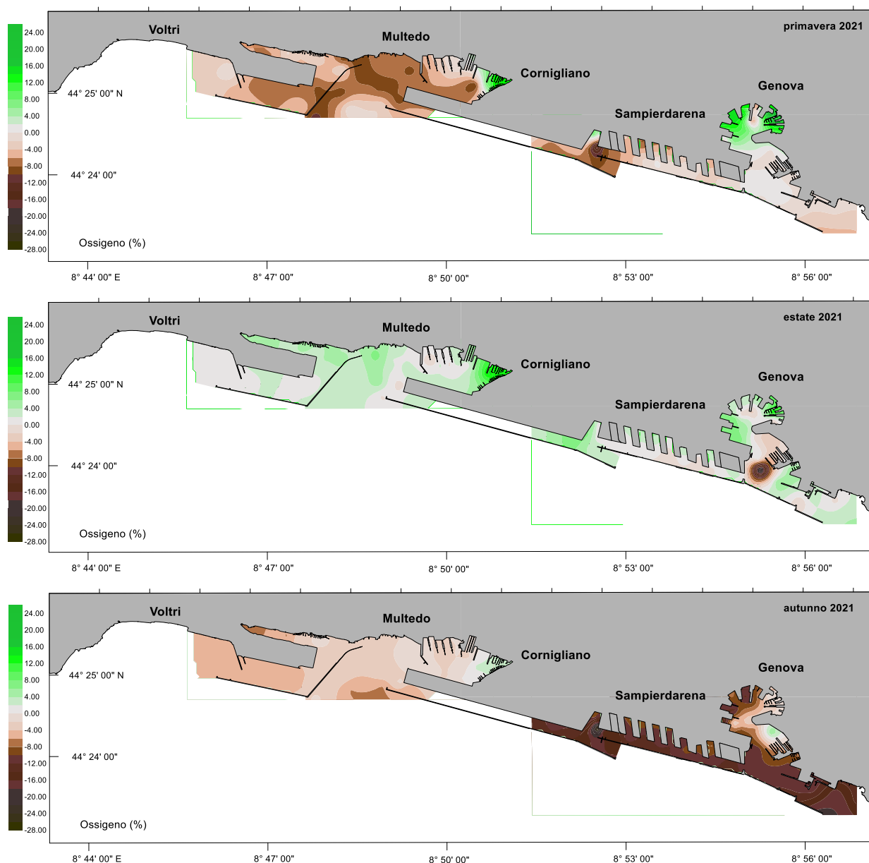
Fig. 3.6 Distribuzione spaziale delle anomalie della percentuale di saturazione dell'ossigeno nel 2021
