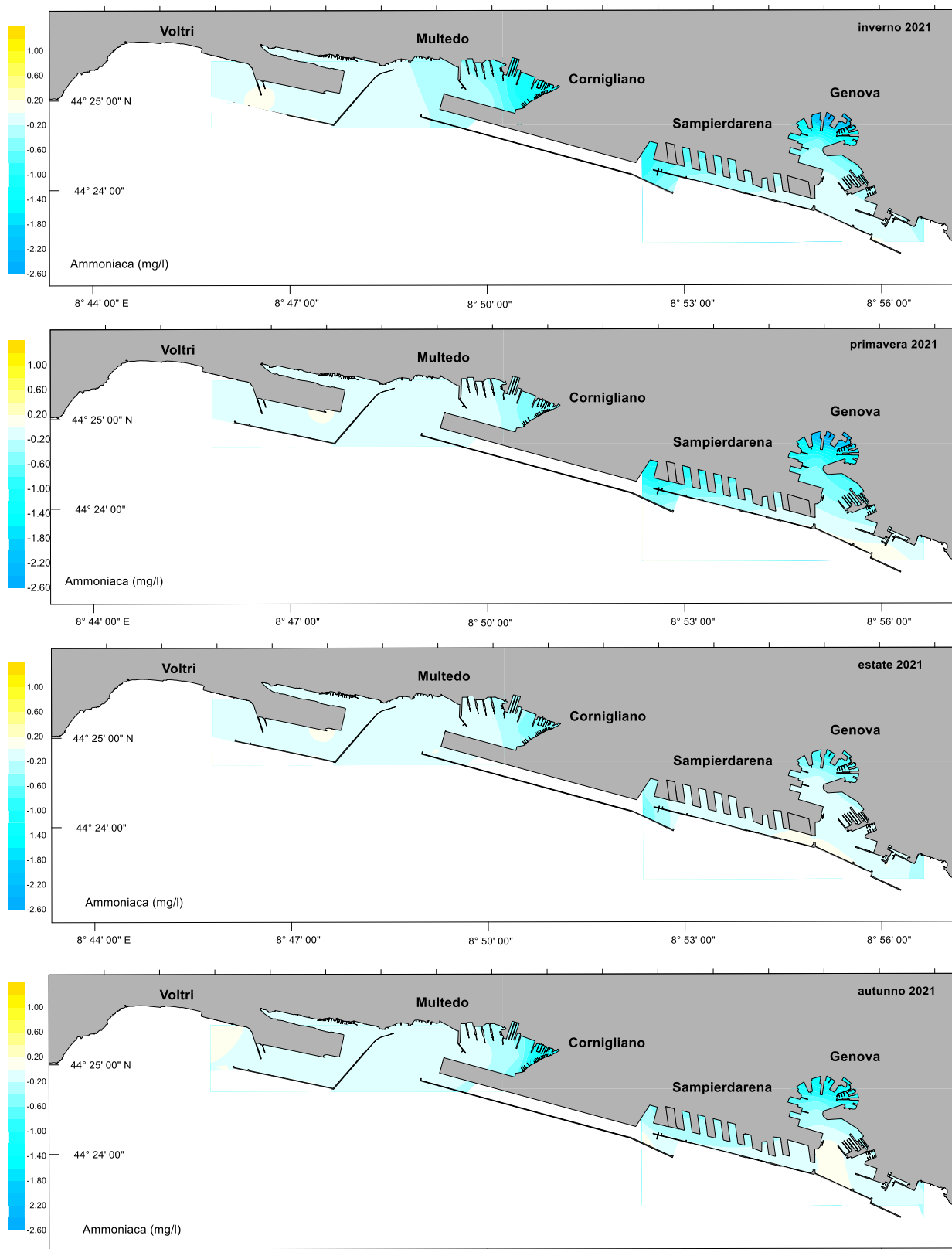
Fig. 3.8 Distribuzione spaziale delle anomalie dell'ammoniaca nel 2021
