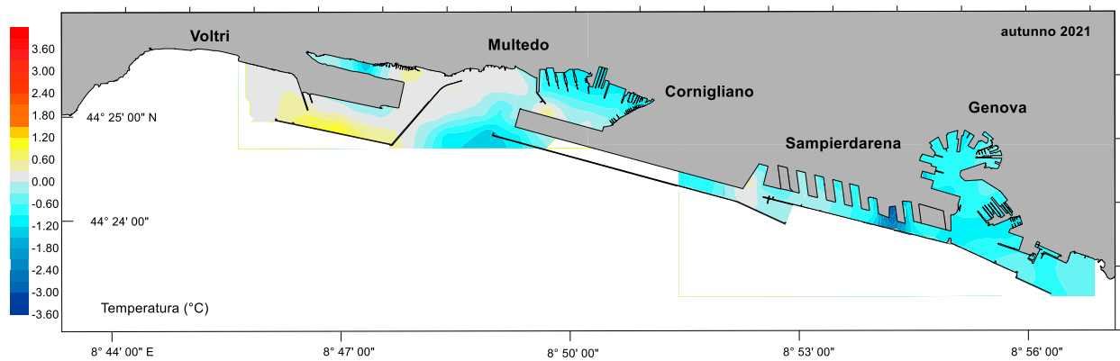
Fig. 3.4 Distribuzione spaziale delle anomalie della temperatura dell'acqua nel 2021
