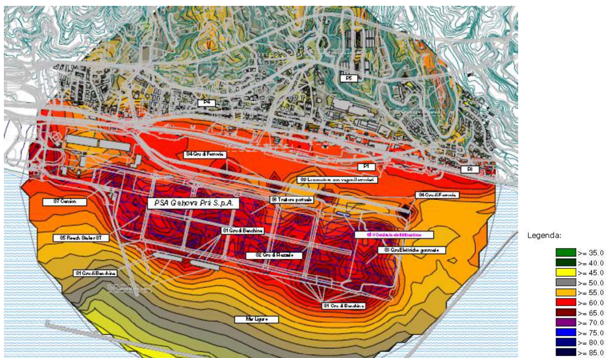
Figura 5.10: Mappa della rumorosità allo stato di progetto in periodo diurno – porto attivo escluso il traffico stradale e ferroviario
