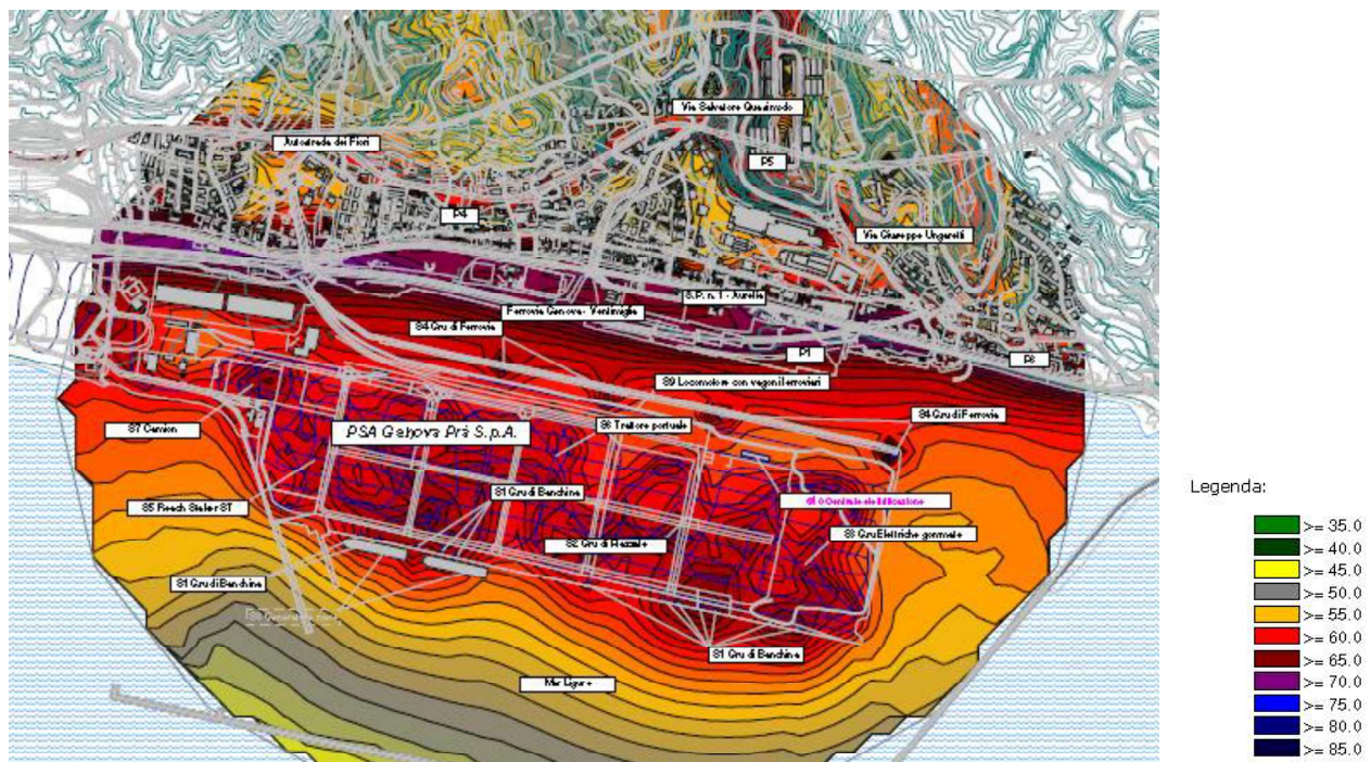
Figura 5.9: Mappa della rumorosità allo stato di progetto in periodo diurno – porto attivo comprensivo del traffico stradale e ferroviario
