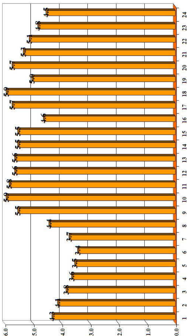
Distribuzione oraria SO 2 (ug/m 3 )
