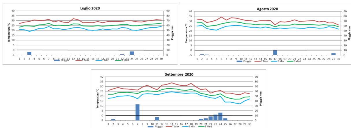
Fig. 1 Andamento delle precipitazioni e della temperatura nei mesi Luglio, Agosto e Settembre 2020 ( http://www.cartografiarl.regione.liguria.it )
